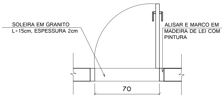
PLANTA-ESQUADRIA P3
