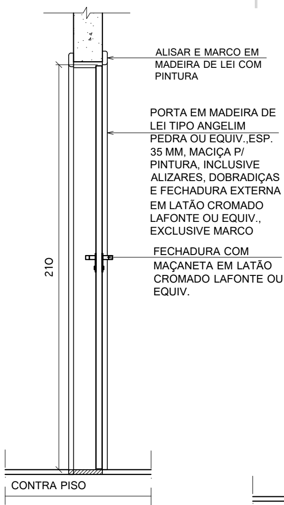
SEÇÃO-ESQUADRIA P2
