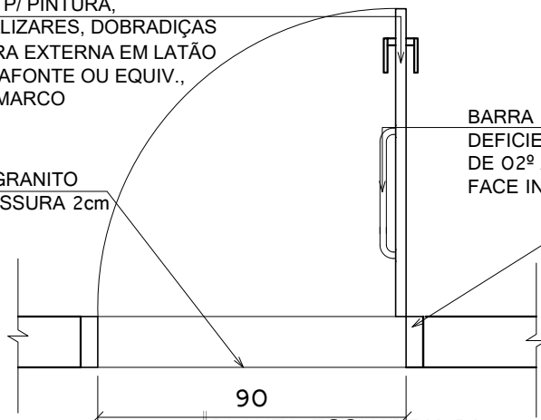
PLANTA-ESQUADRIA P1
