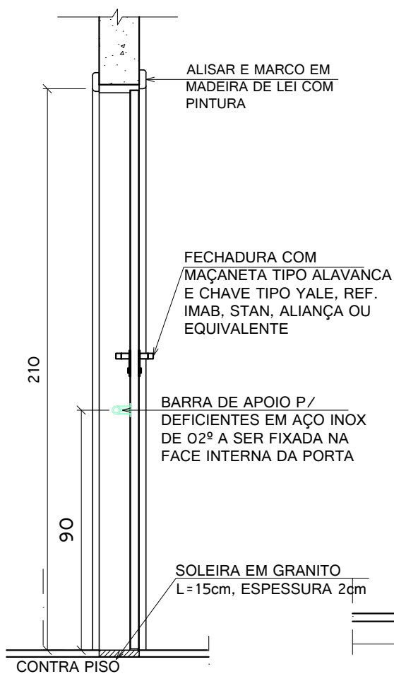
SEÇÃO-ESQUADRIA P1
