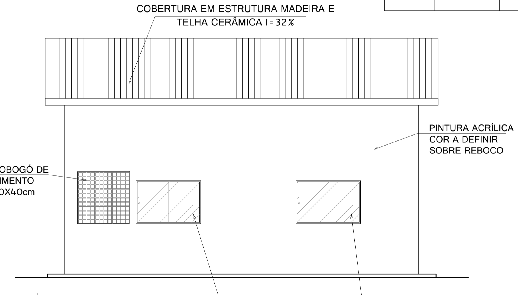
FACHADA LAT.ESQ. ESC.:1/50
