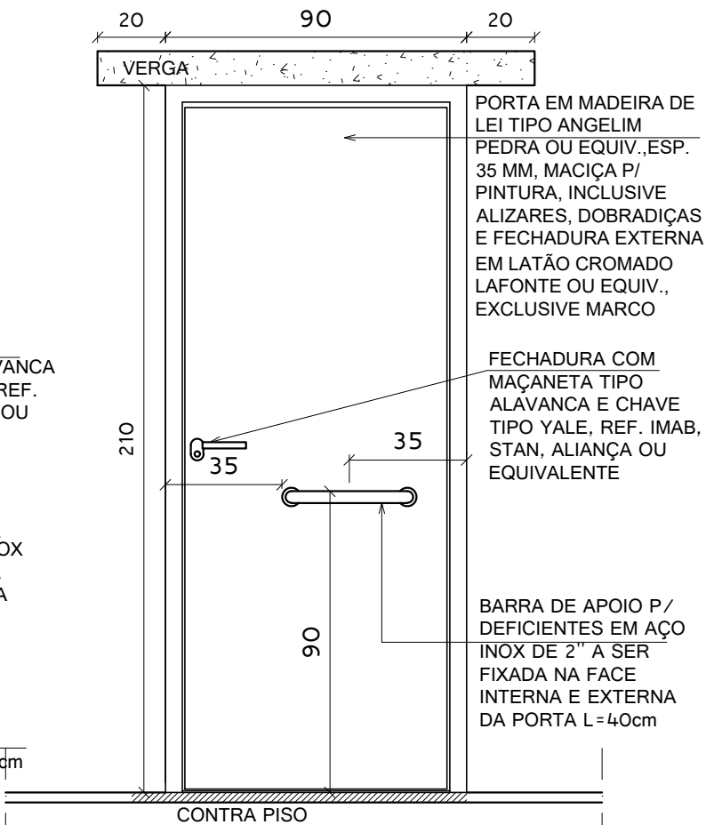
VISTA-ESQUADRIA P1
