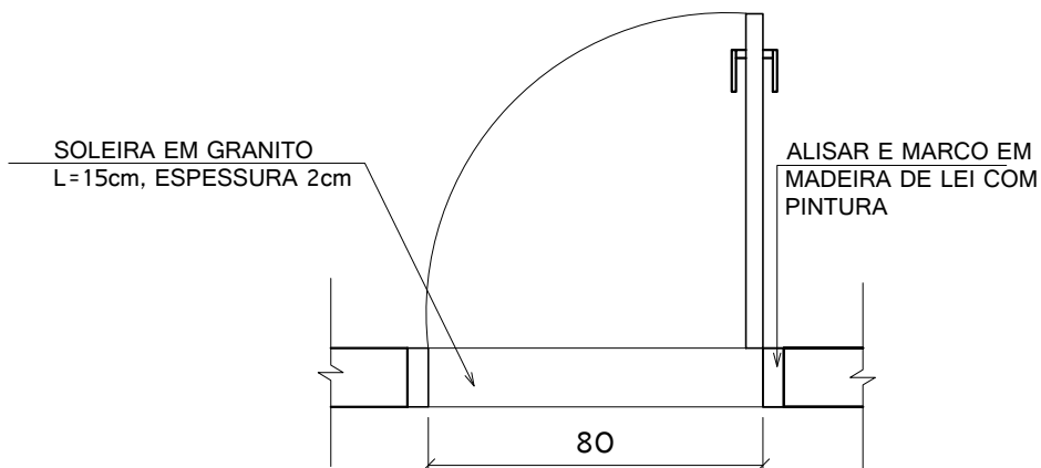
PLANTA-ESQUADRIA P2
