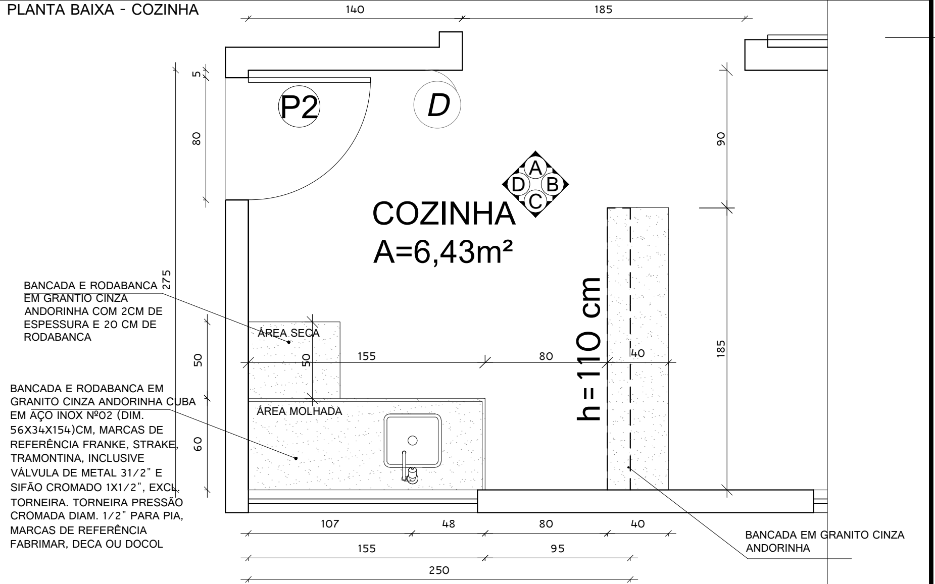
PLANTA BAIXA COZINHA ESC: 1/25
