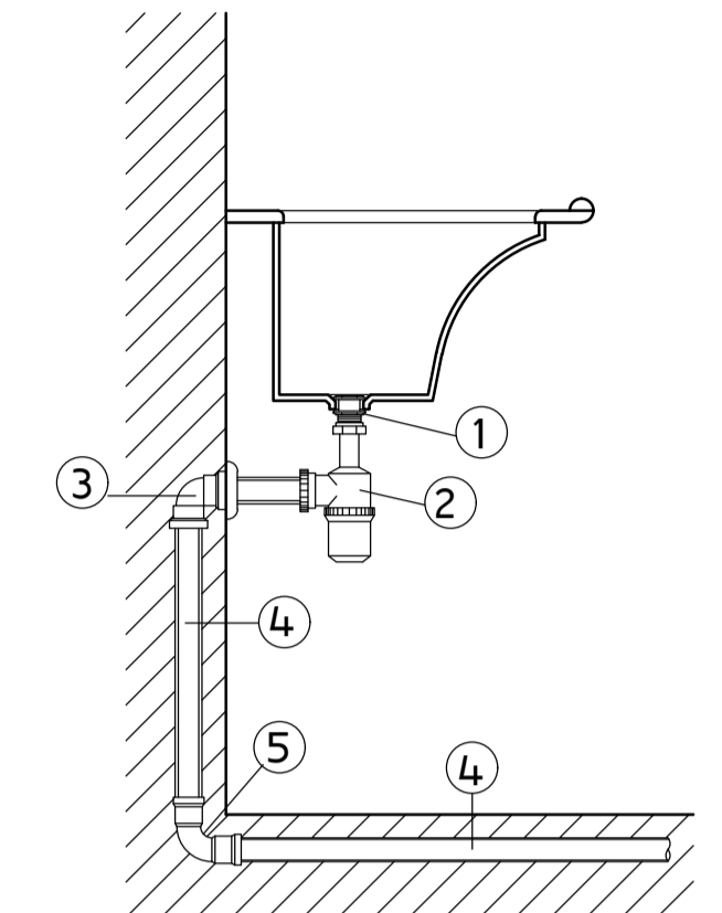
DETALHE TANQUE SEM ESCALA
