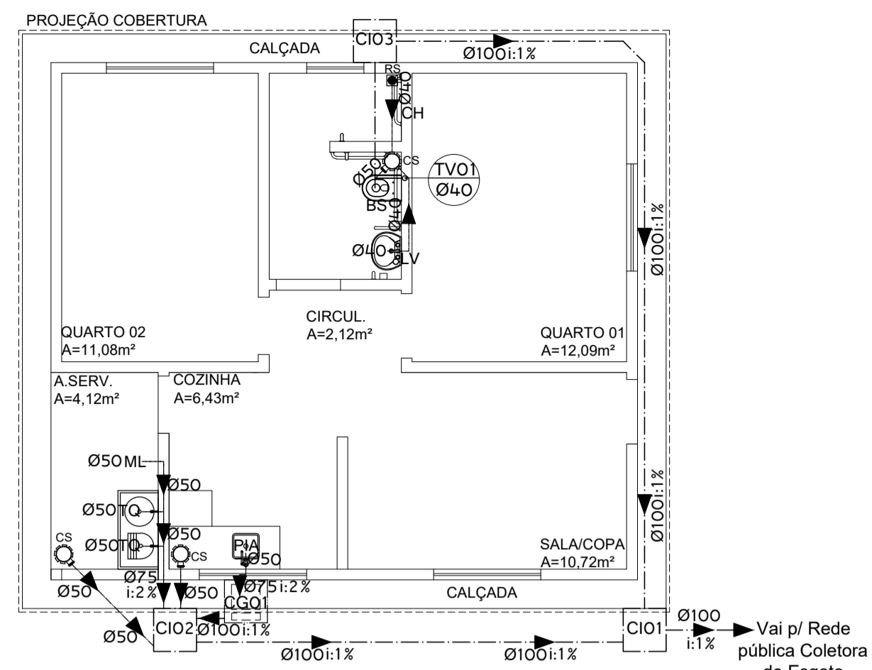
PLANTA BAIXA ESGOTO ESC: 1/75
