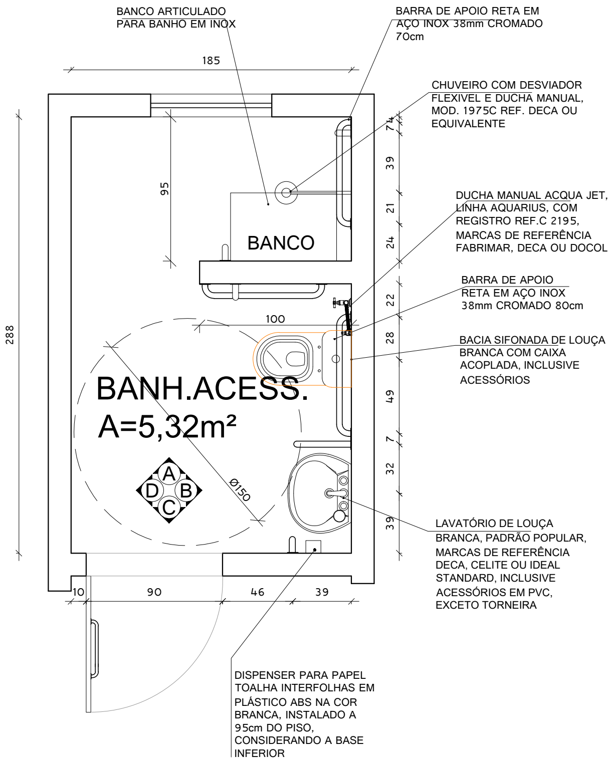
PLANTA BAIXA BAN. PCD FEM. MASC. ESC: 1/25
