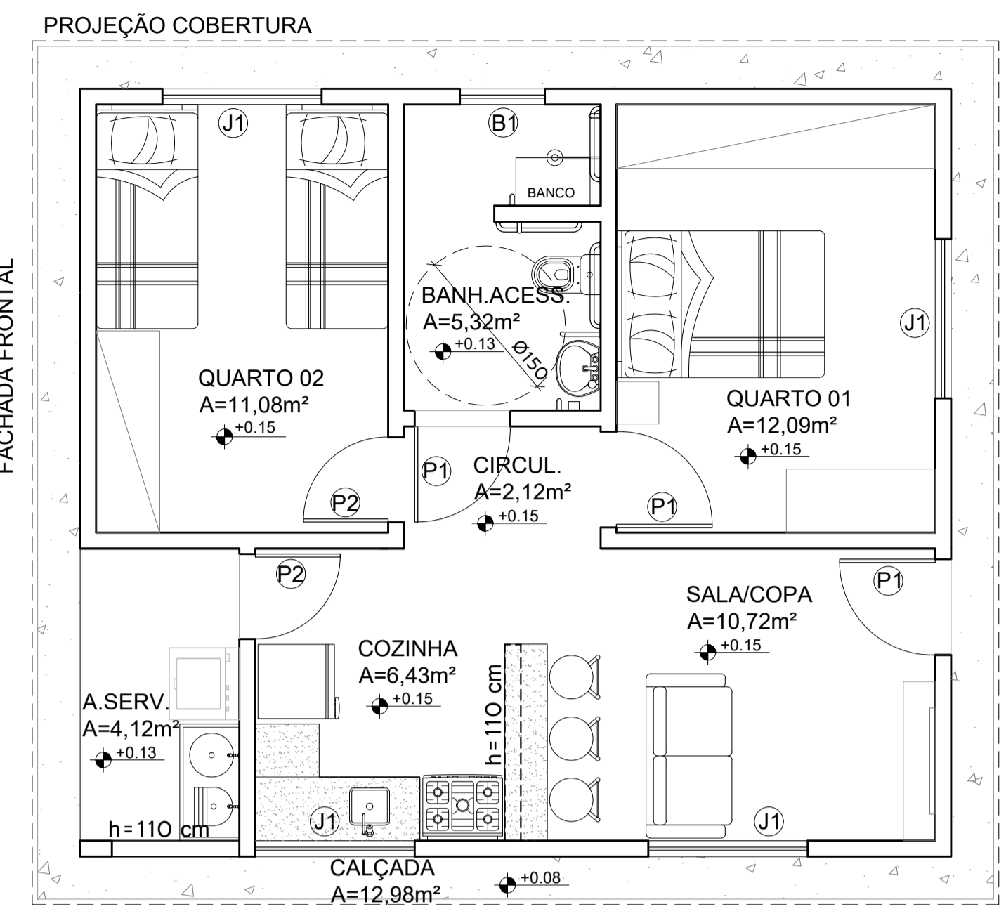
LAYOUT ESC.:1/50
