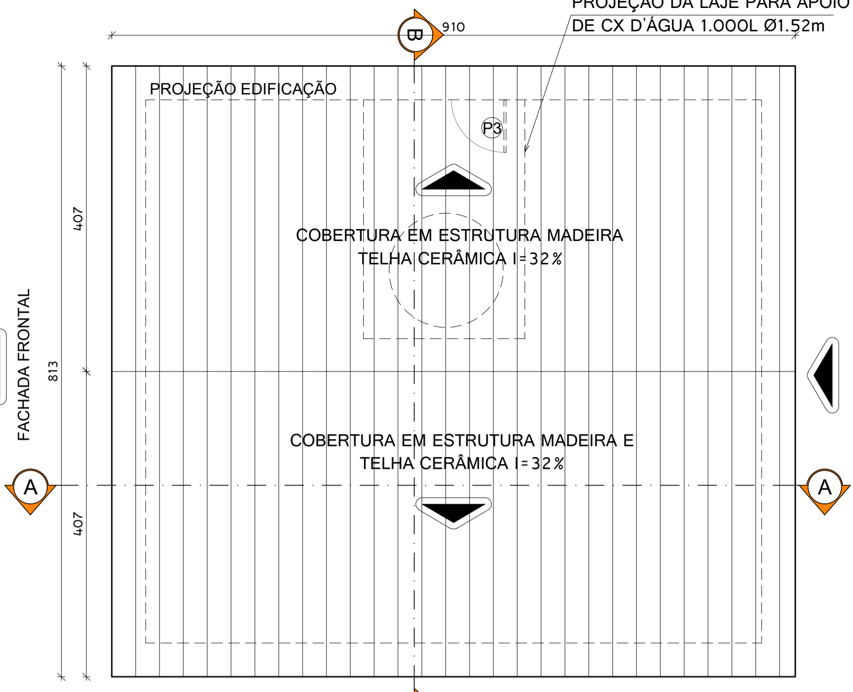
COBERTURA ESC.:1/50
