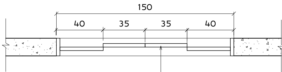
PLANTA-ESQUADRIA J1
