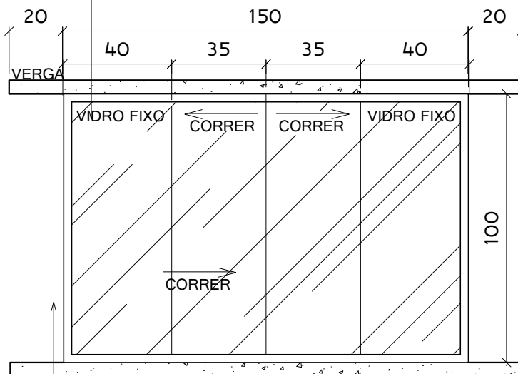
VISTA-ESQUADRIA J1
