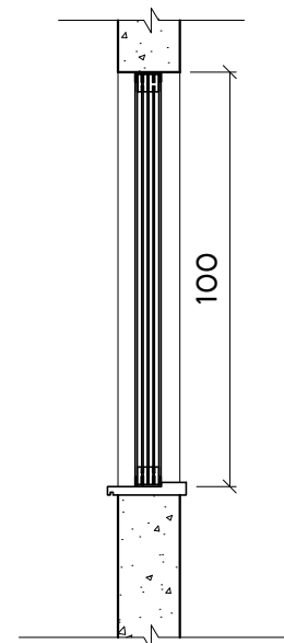
SEÇÃO-ESQUADRIA J1
