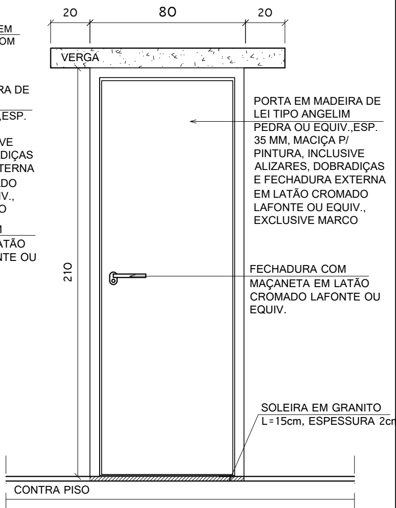
VISTA-ESQUADRIA P2
