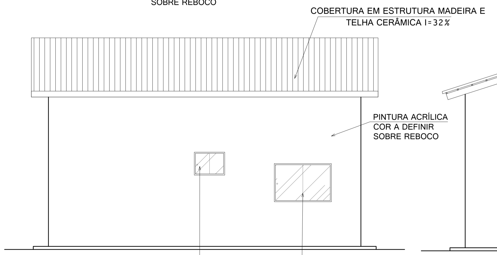
FACHADA LAT.DIR. ESC.:1/50
