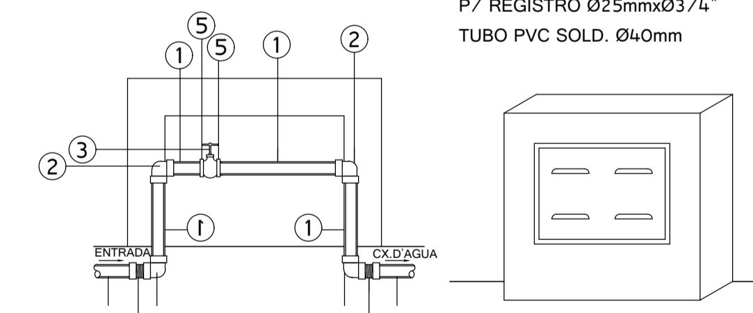
DETALHE DE LIGAÇÃO DE HIDRÔMETRO PARA RESERVATÓRIO SEM ESCALA
