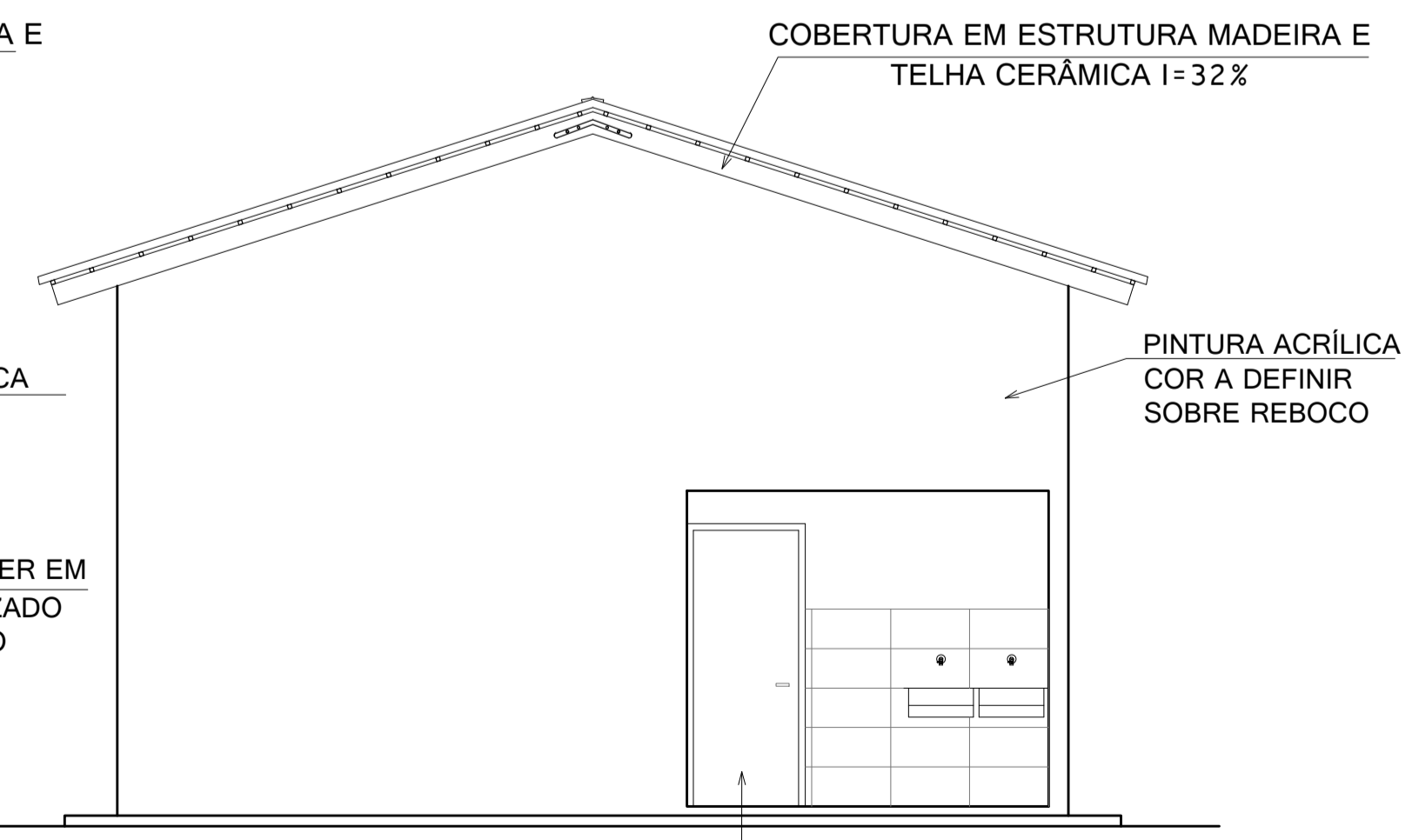
FACHADA FUNDOS ESC.:1/50
