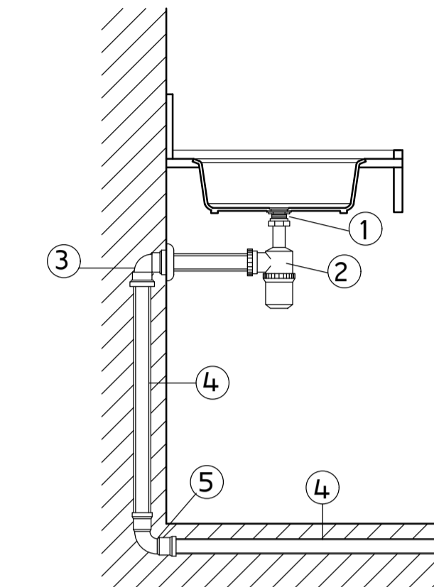
DETALHE LIGAÇÃO DE PIA SEM ESCALA
