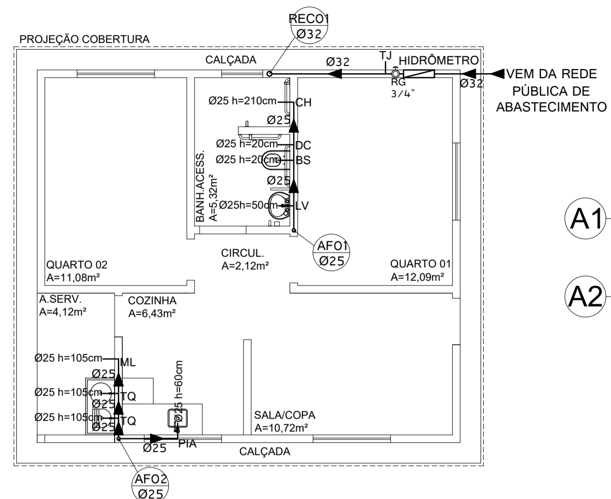
PLANTA BAIXA ÁGUA FRIA ESC: 1/75
